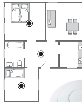
Installation von Rauchwarnmeldern am Beispiel einer Drei-Zimmer-Wohnung.
