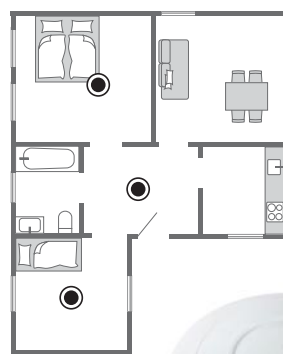
Installation von Rauchwarnmeldern am Beispiel einer Drei-Zimmer-Wohnung.
